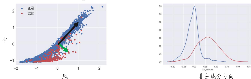
图 3-30：风速与功率非主成分方向投影特征
