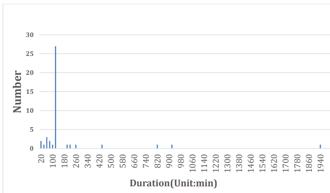
图 3-15: 结冰故障持续时间统计
