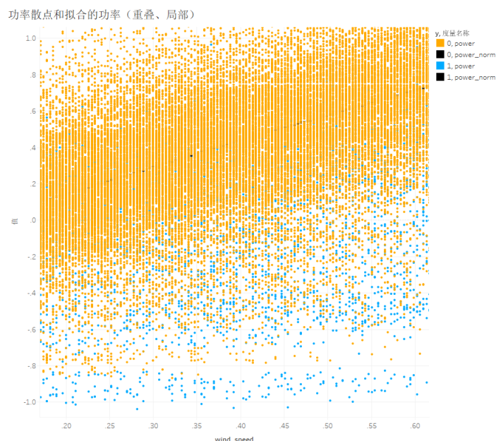
图 3-9：风速-功率散点和拟合的功率
