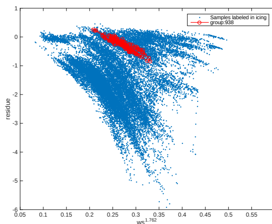
图 2-7：一个周期内结冰数据的分布
