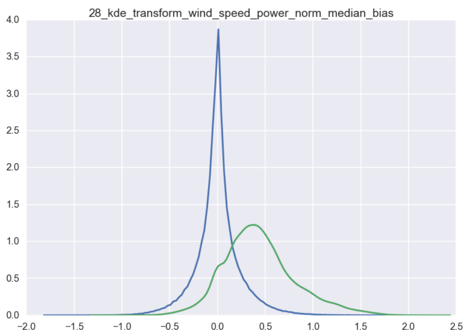
图 3-14：风速-功率拟合曲线与实际功率的残差的核密度分布图 (蓝色为不结冰数据，基本分布在 0 的附近，而且非常集中。
