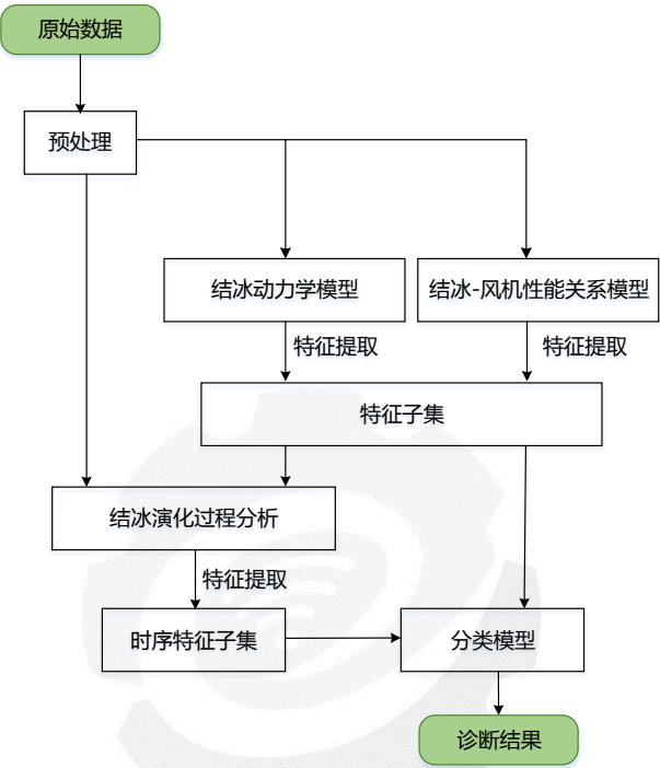
图 2-3：风机叶片结冰预测分析流程
