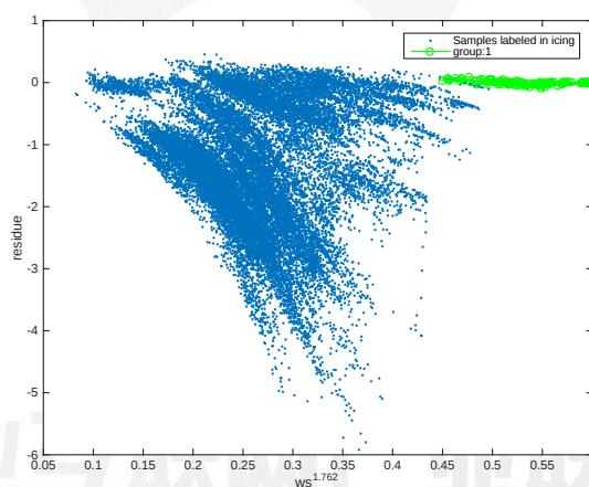
图 2-8：一个时间周期内非结冰数据的分布
