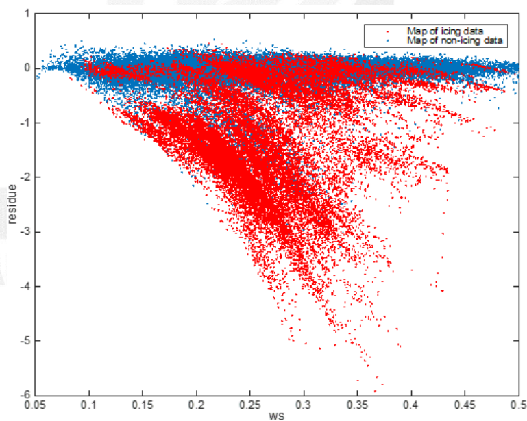
图 2-5: 结冰质量—风速关系
