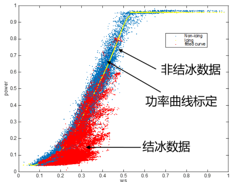
图 2-4: 功率特性线拟合
