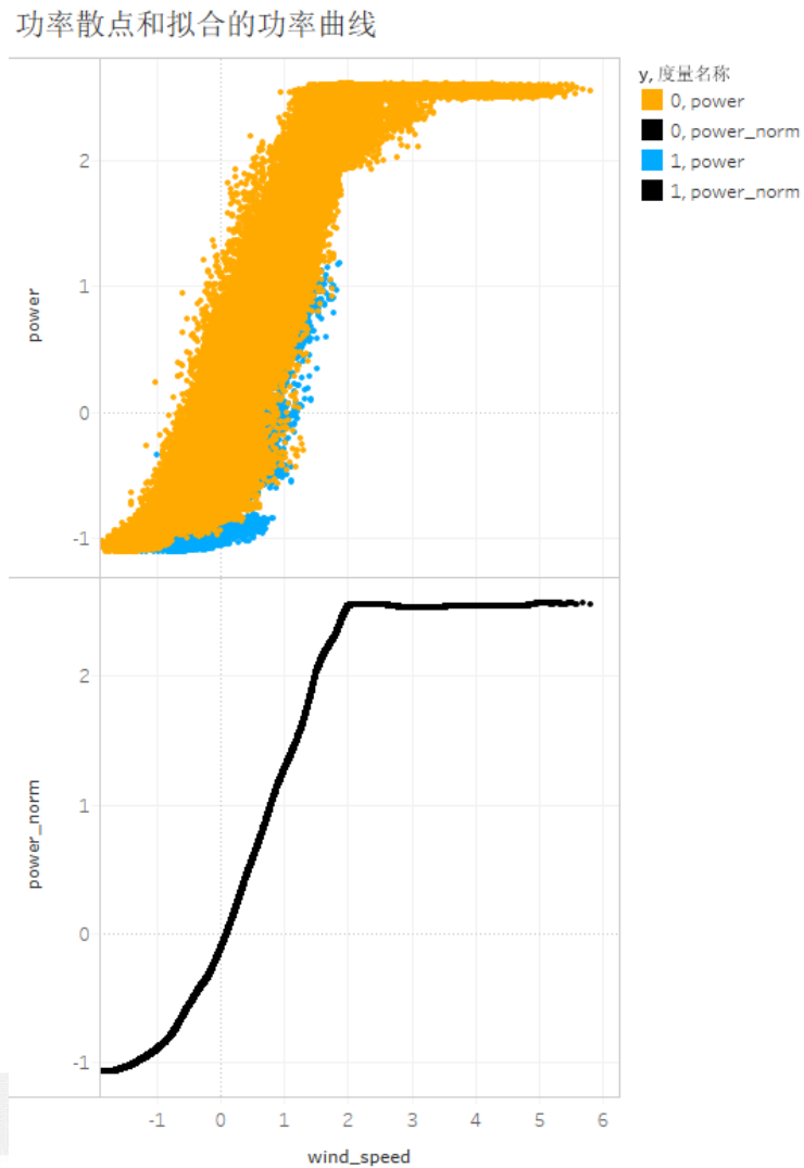
图 3-8：风速-功率散点图
