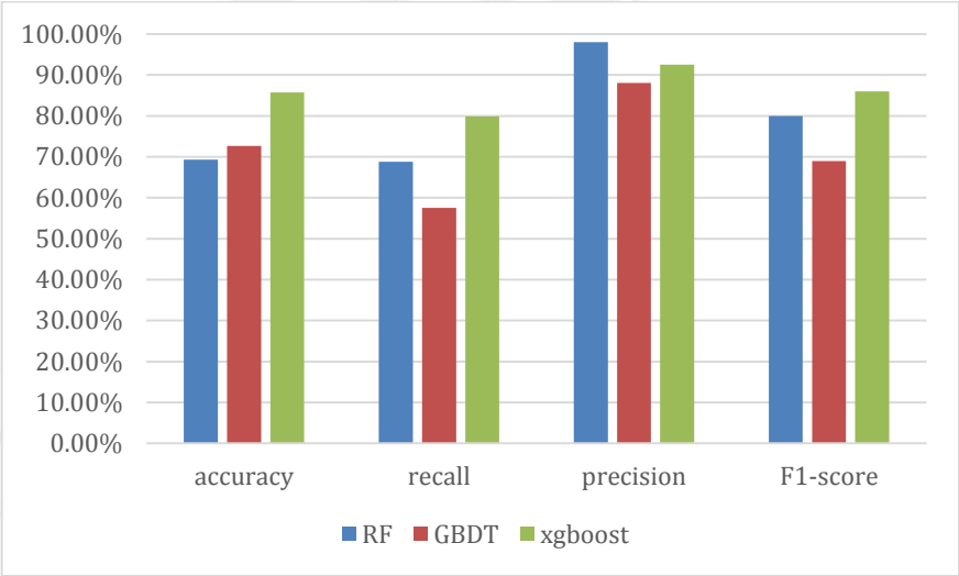
图 3-22：RF、GBDT、XGBoost 三种基分类器在不同评价指标下的比较
