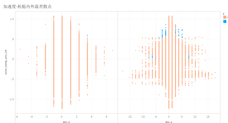
图 3-13：加速度-机舱内外温差散点
