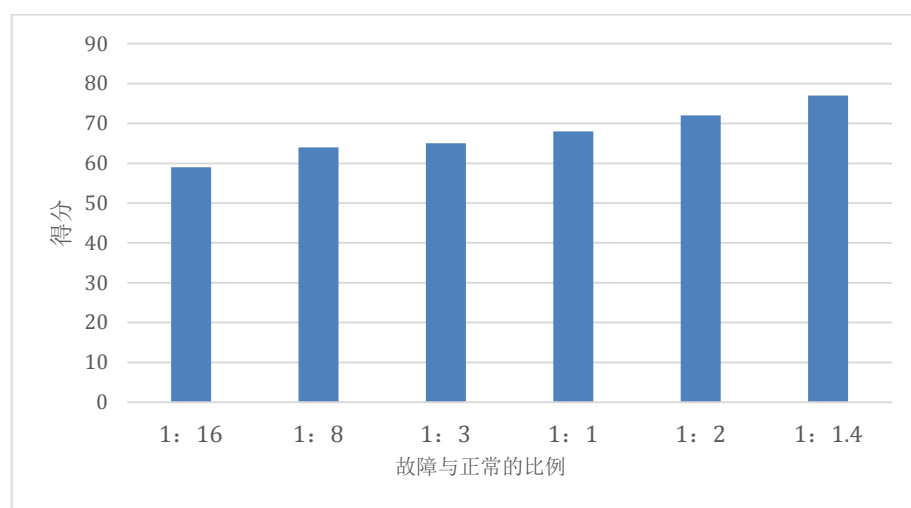
图 3-23: 不同故障与正常样本个数比例下的验证集得分
