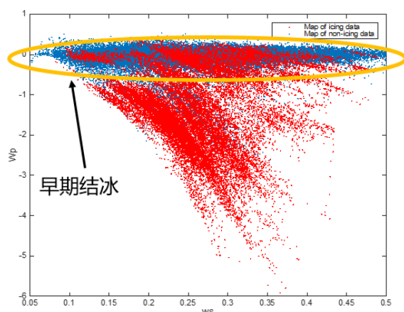
图 2-6：早期结冰数据
