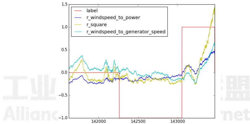
图 3-3：特征组合波形
