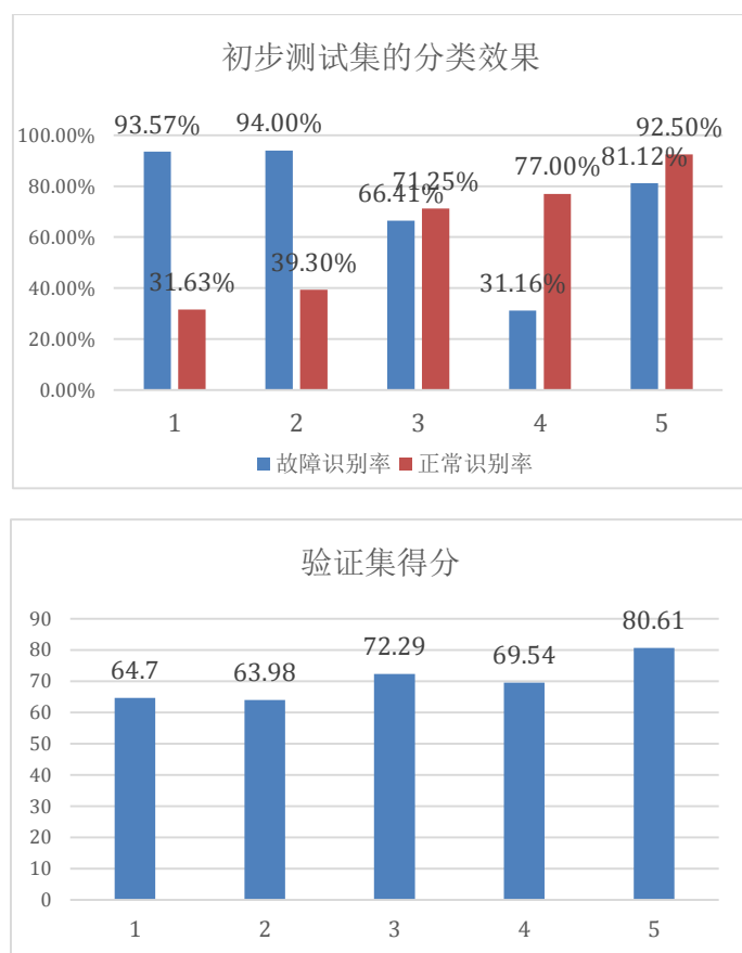
图 3-24: 交叉验证在初步测试集和验证集上的结果
