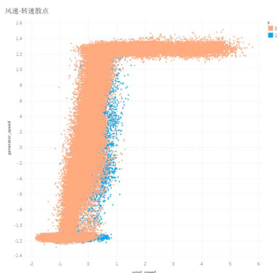
图 3-10：风速-转速散点图
