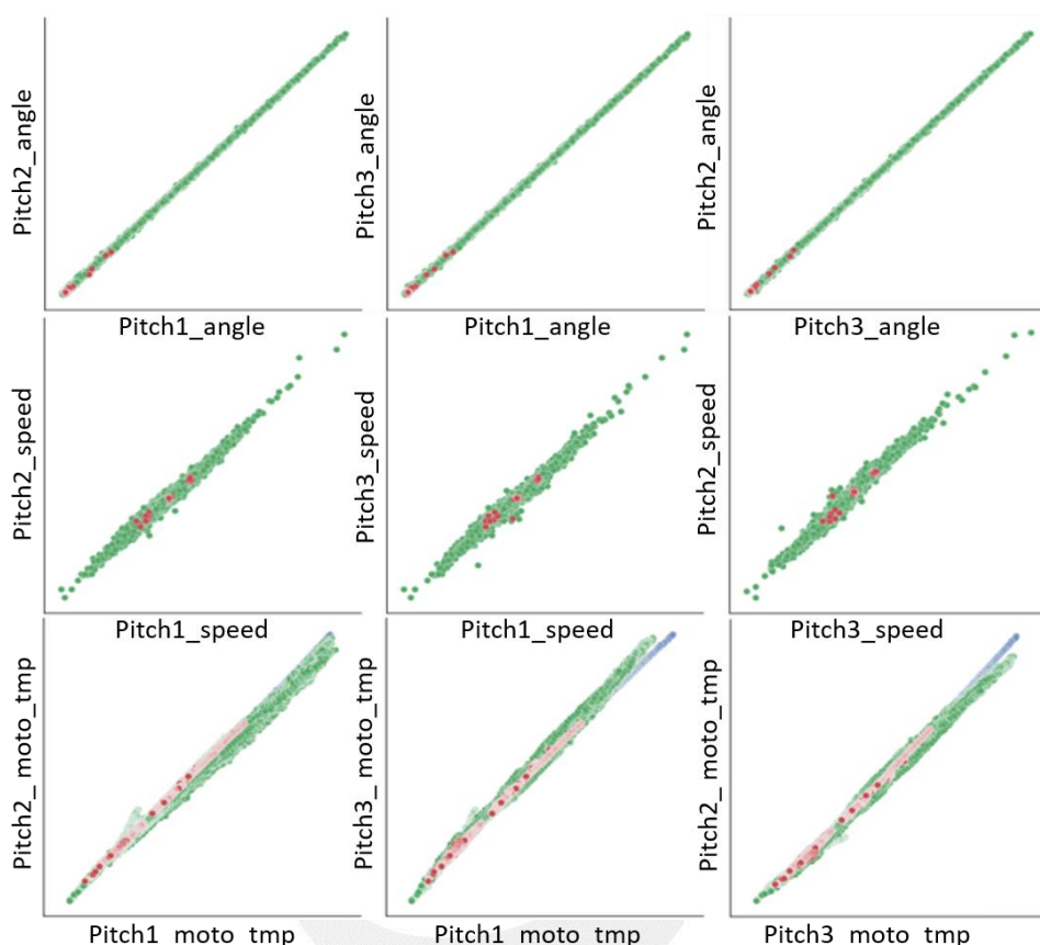
图 3-2: 叶片角度、速度、变桨电机温度数据分布
