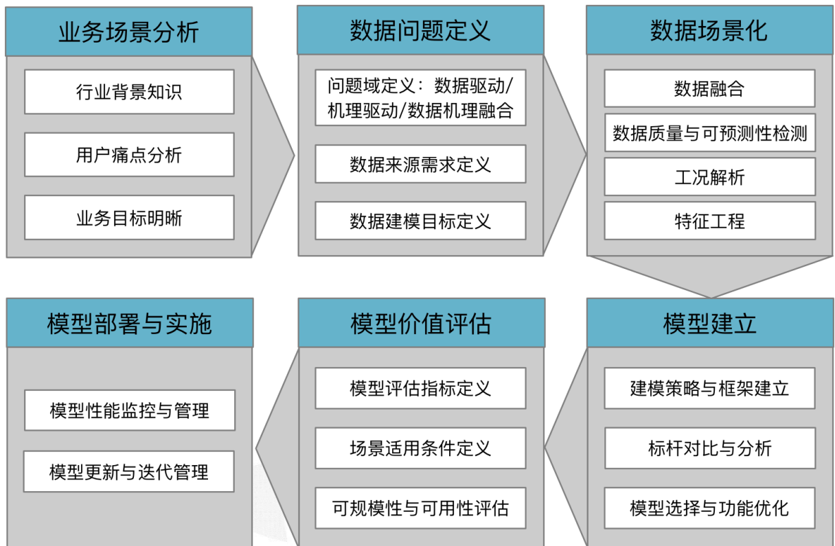
图 2-2：工业大数据的建模过程
