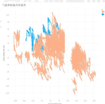
图 3-11：气温和机舱内外温差
